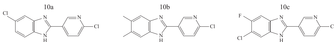
Рис. 6. Структура производных бензимидазола, взаимодействующих с каналами KV7
