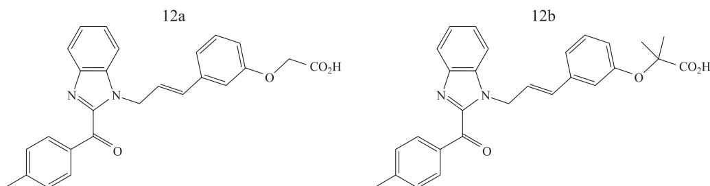
Рис. 8. Структура производных бензимидазола, взаимодействующих с рецептором, активируемым пероксисомным пролифератором гамма (PPAR \gamma )
