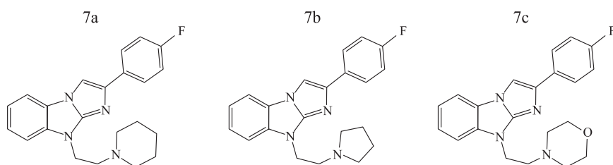
Рис. 3. Структура производных бензимидазола, взаимодействующих с КОР
