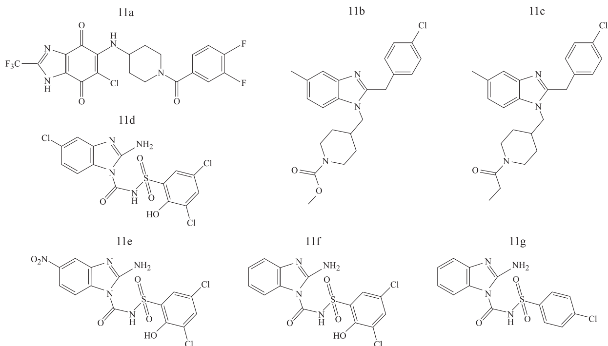
Рис. 7. Структура производных бензимидазола, взаимодействующих с пуриновыми рецепторами
