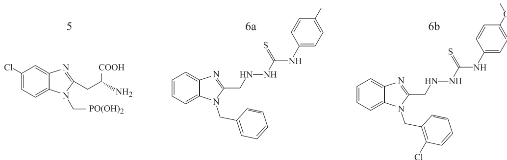
Рис. 2. Структура производных бензимидазола, взаимодействующих с глутаматными рецепторами
