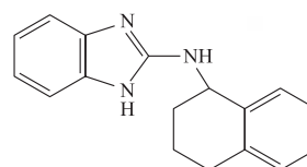
Рис. 5. Структура производного бензимидазола, взаимодействующего с TRPM7
