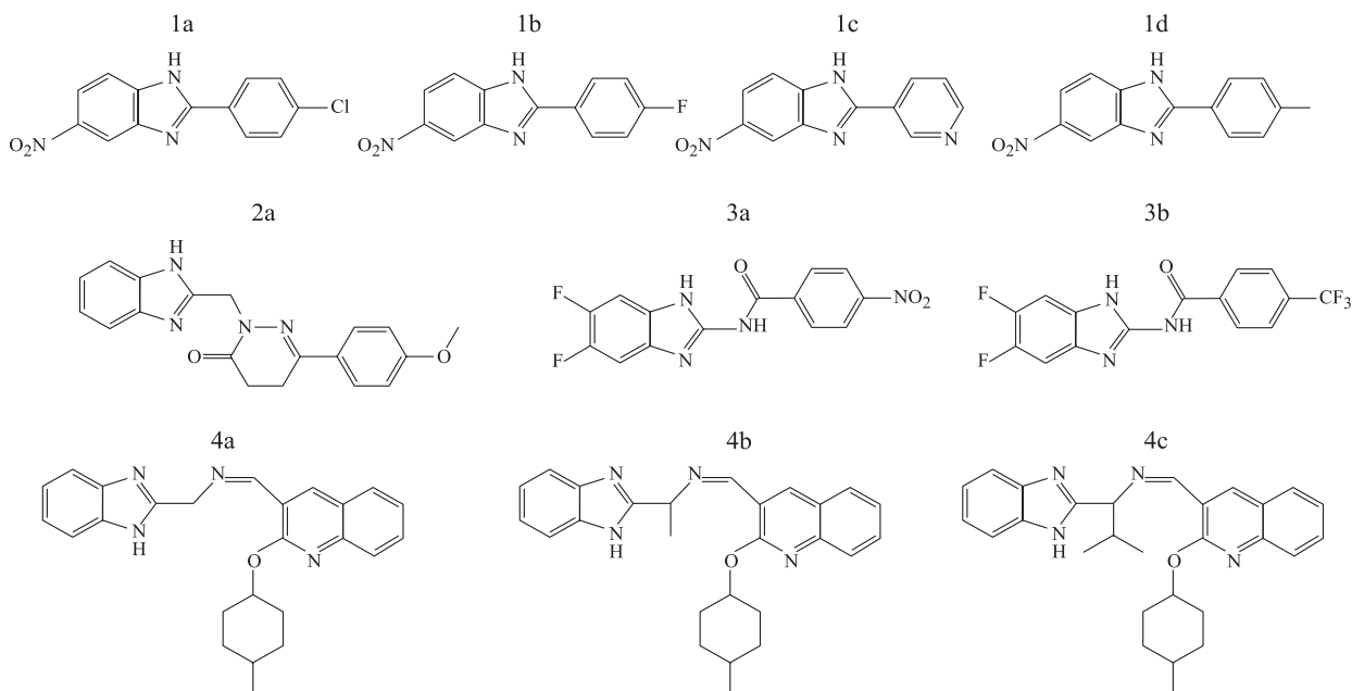
Рис. 1. Структура производных бензимидазола, взаимодействующих с рецепторами ГАМК
