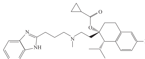
Рис. 4. Структура производного бензимидазола, взаимодействующего с кальциевыми каналами Т-типа
