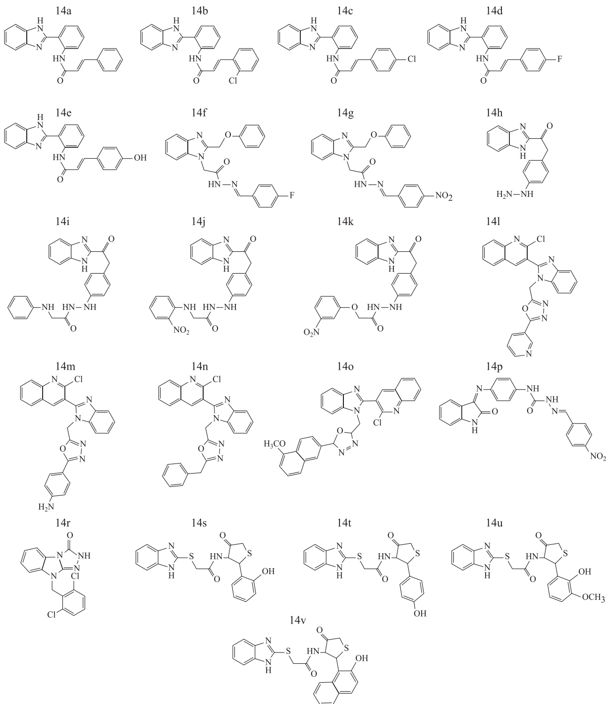
Рис. 10. Структура производных бензимидазола, противосудорожный механизм действия которых не установлен Fig. 10. Structures of benzimidazole derivatives, the mechanism of anticonvulsant action of which has not been established
