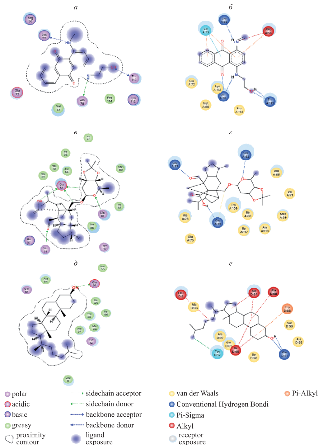
Рис. 3. Двумерная визуализация молекулярных взаимодействий СТВ с GM1 (а, б), GM3 (в, г), холестерином (д, е); а, в, д – интерпретация в Molecular Operating Environment, б, г, е – интерпретация в Discovery studio Fig. 3. Two-dimensional visualization of molecular interactions of cholera toxin subunit B with GM1 (a, б), GM3 (в, г), холестерином (д, е); а, в, д – interpreted in Molecular Operating Environment, б, г, е – interpreted in Discovery Studio
